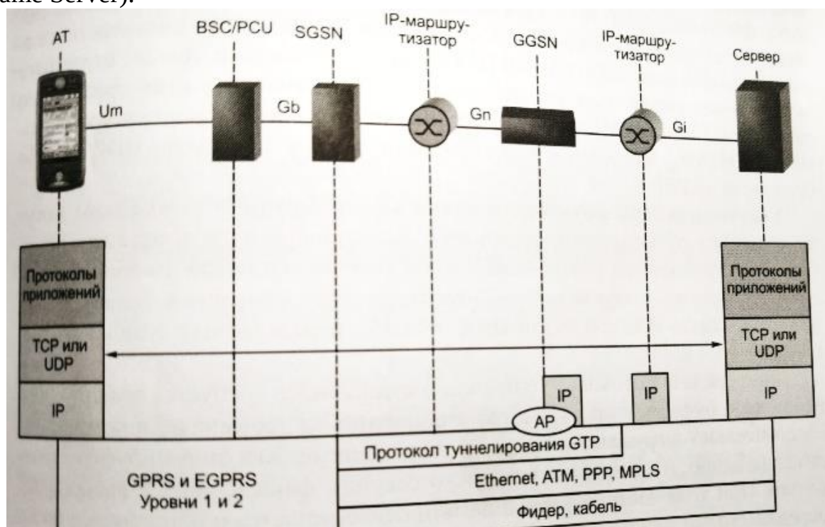
Рис.3.14. Передача IP-пакетов в подсистеме GPRS
