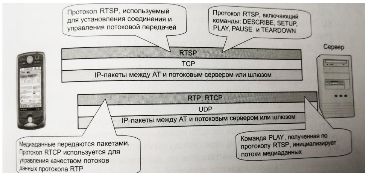
Рис.3.15 Использование IP протокола для передачи потокового аудио/видео.
