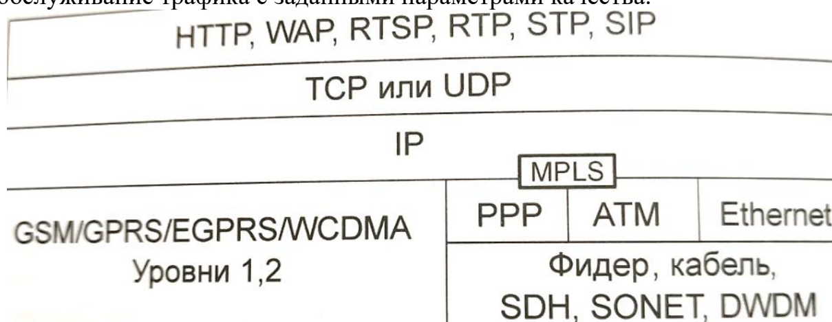
Рис.3.13. Многоуровневая архитектура протокола в сети GPRS/UMTS
