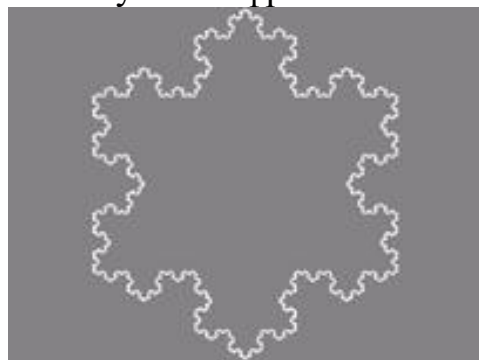
Рисунок 2. Снежинка Коха Серпинского
