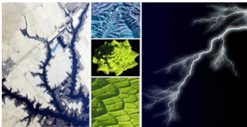
Рисунок 6. Природные фракталы
