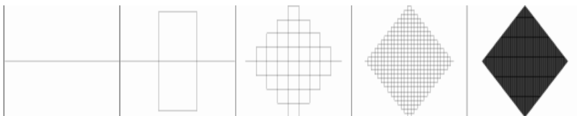
Рисунок 1. Пыль Кантора
