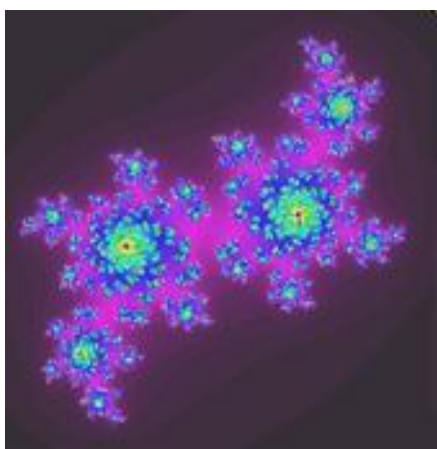
Рисунок 4. Множество Жюлиа Рисунок 5. Множество Мандельброта
